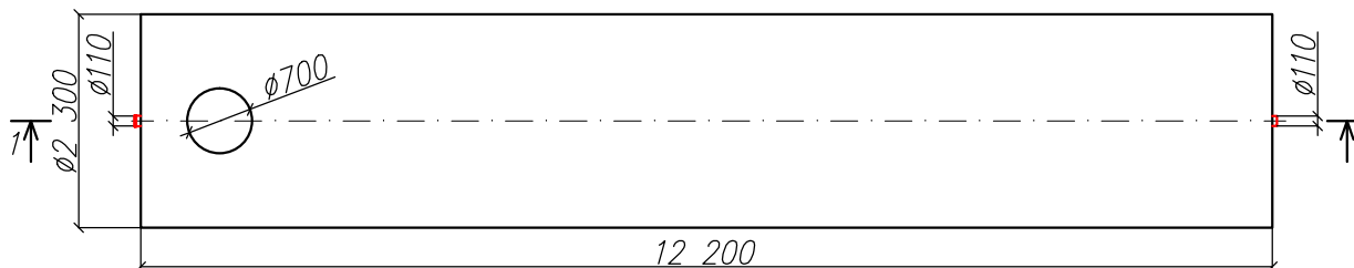
Вид сверху
