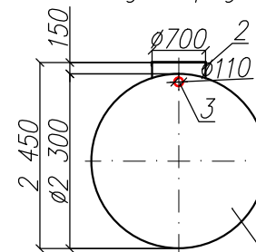
Вид спереди
