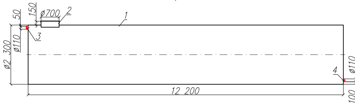
Разрез 1-1
